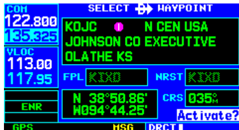
Figure 1-27 'Activate?' Highlighted
